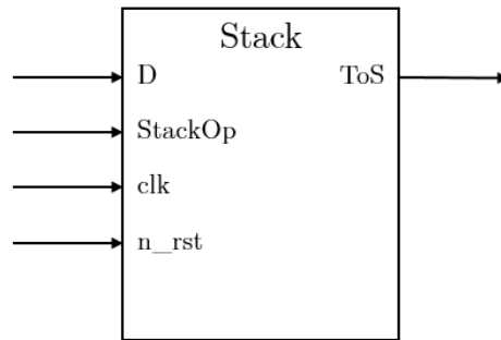
Figur 3.1: Symbol av stacken som ska implementeras. Anslutningarna D och ToS är 6 bitar breda och StackOp 2 bitar bred.
