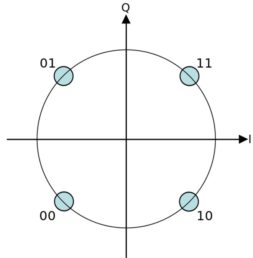
Konstellationsdiagram
