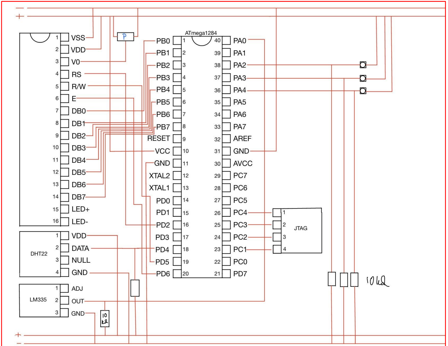
Figur 2: väderstationens krettschema
